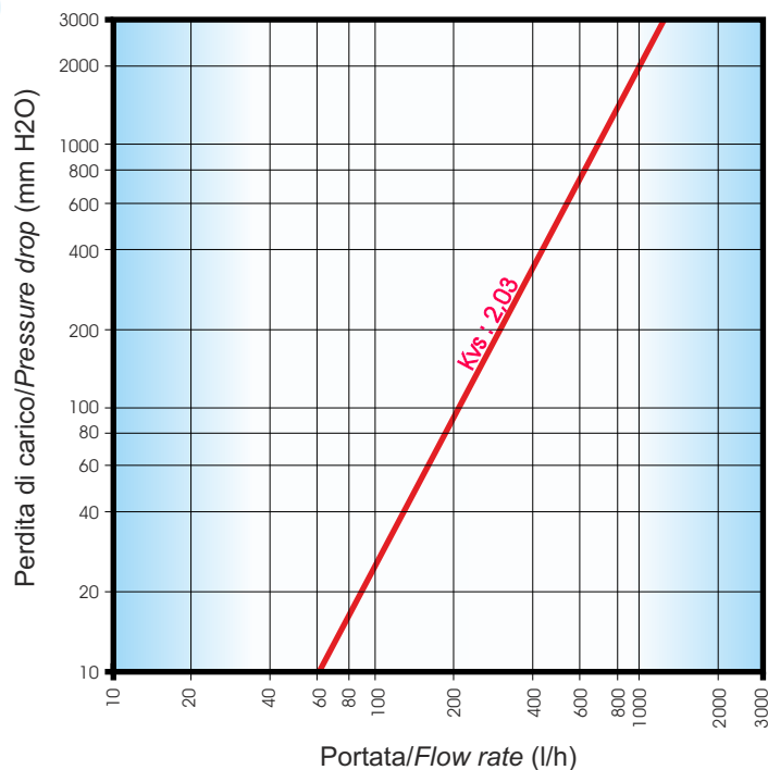
Diagramma perdite di carico Pressure loss diagram
